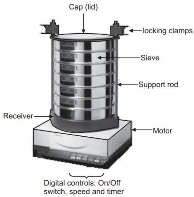
Fig: Sieve Shaker
