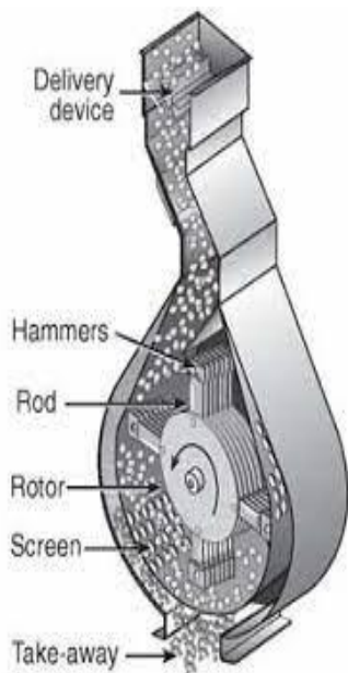
Fig: Hammer Mill
